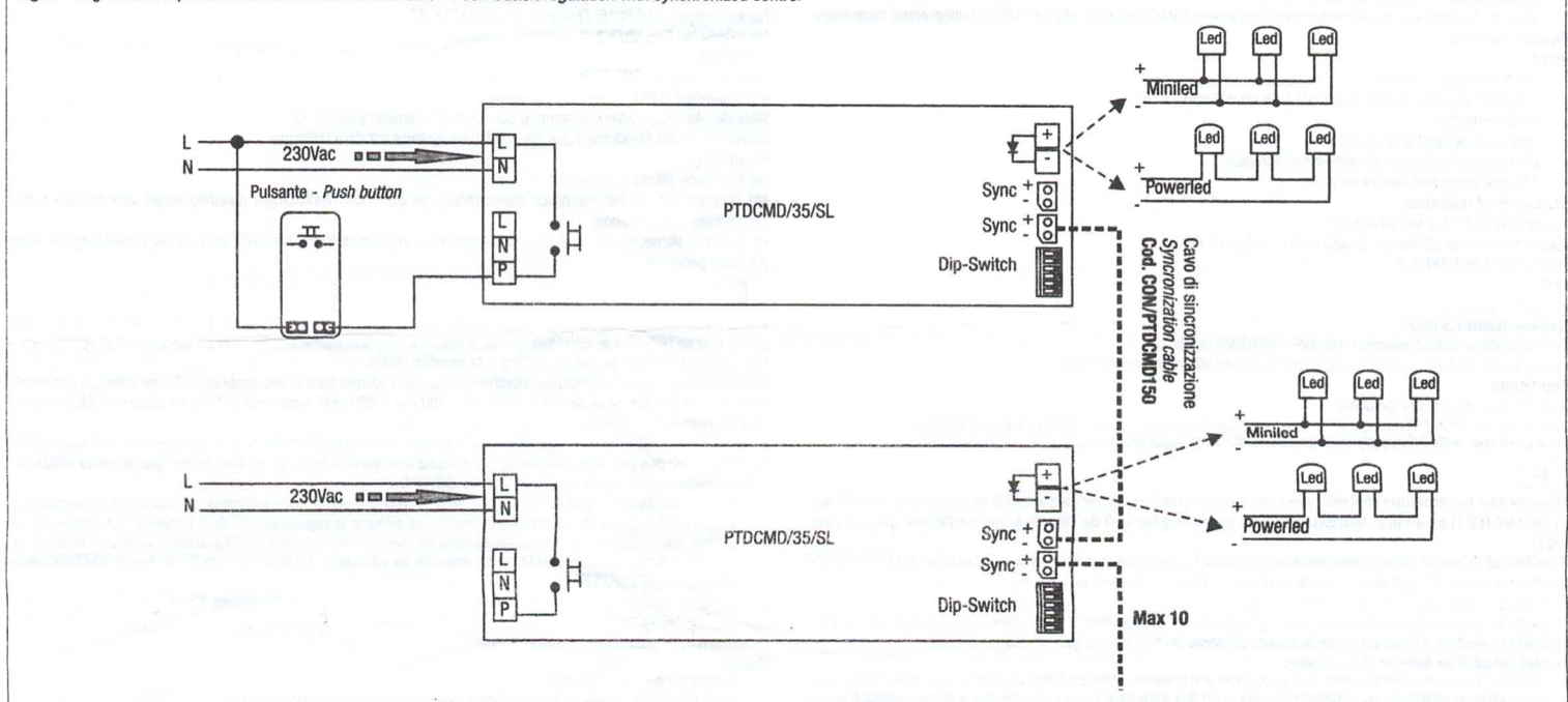
Fig. 3 - Regolazione a pulsante con comando sincronizzato - Push-button regulation with synchronized control
