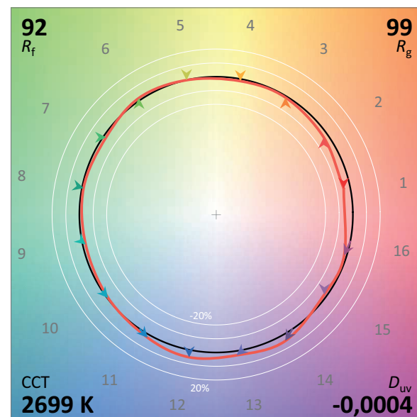
Farbvektordiagramm
