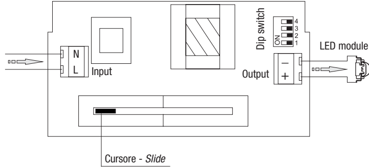
Fig. 1 - Schema di collegamento - Wiring diagram
