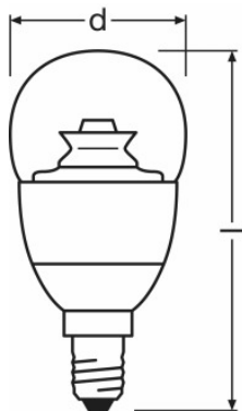
PARATHOM CL P 40 ADV 6 W/827 E14 CS
