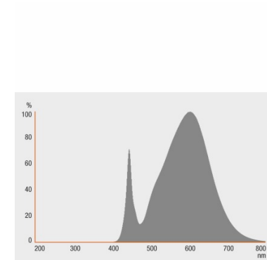
PARATHOM CL P 25 ADV 4 W/827 E14 CS, PARATHOM CL P 25 ADV 4 W/827 E27 CS, PARATHOM CL P 25 ADV 4 W/827 E14 FR, PARATHOM CL P 25 ADV 4 W/827 E27 FR
