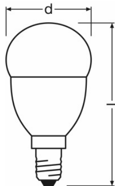
PARATHOM CL P 40 ADV 6 W/827 E14 FR
