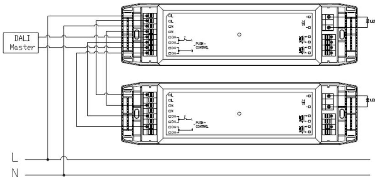
Fig. C: DALI Dimming
