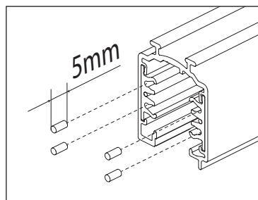
Abb. 5 Mindestlänge Kürzung Pic. 5 Minimum recessing
