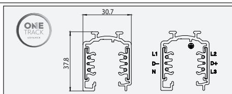
Oberfläche/Aufhängung Schiene (9000A-...-ST) Surface/supended track (9000A-...-ST)
