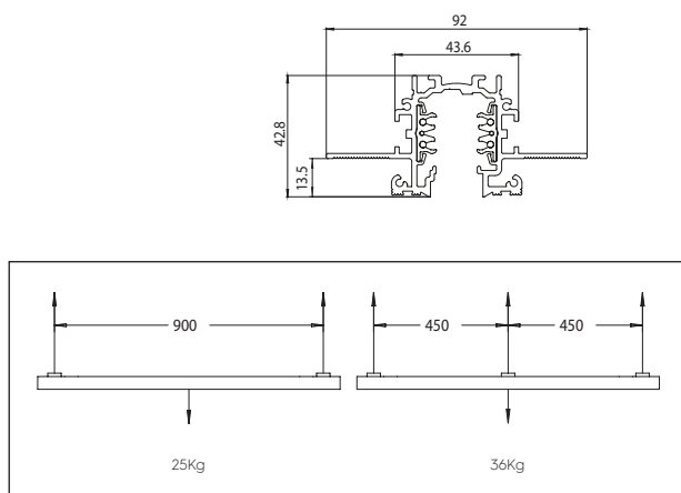
Tragfähigkeit Load scheme
