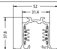
Oberfläche/Aufhängung Schiene (9000A-...-ST) Surface/supended track (9000A-...-ST)
