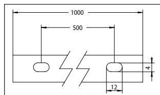
Position der Schlitzlöcher Mounting holes position
