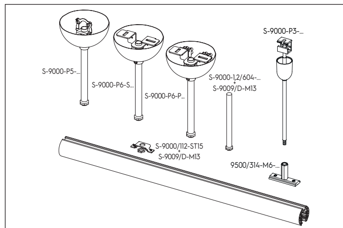
Starre Aufhängungssätze Rigid suspension sets
