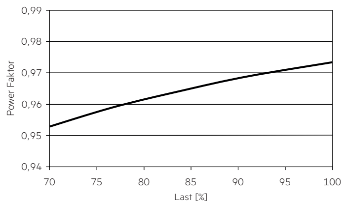
4.1.2 Power Factor in Abhängigkeit von der Last
