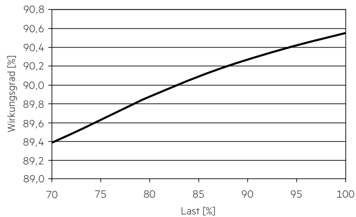
4.3.1 Wirkungsgrad in Abhängigkeit von der Last
