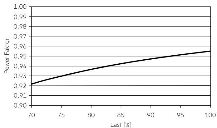
4.3.2 Power Faktor in Abhängigkeit von der Last
