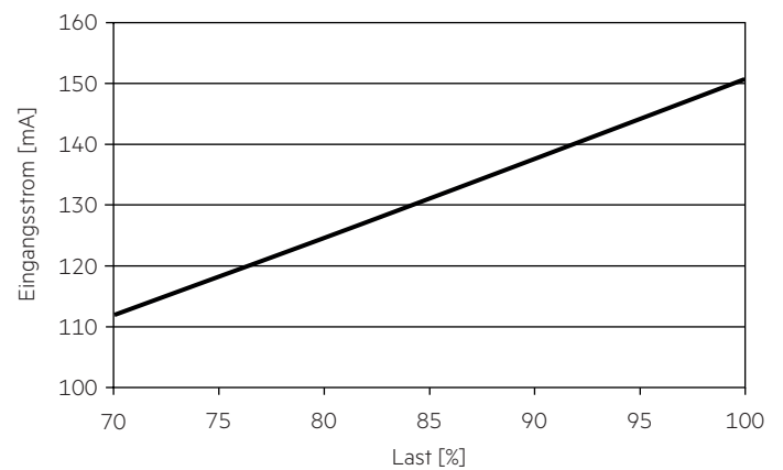
4.3.4 Eingangsstrom in Abhängigkeit von der Last
