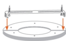
Deckenmontage (direkt)
